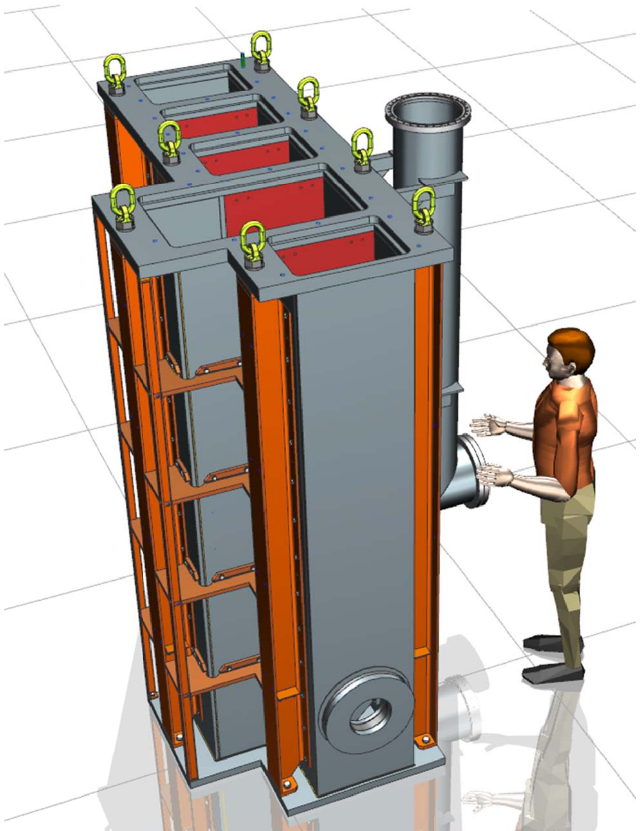
Concept CAD model (15-03-2017) Alleen ter informatie, niet voor productie
